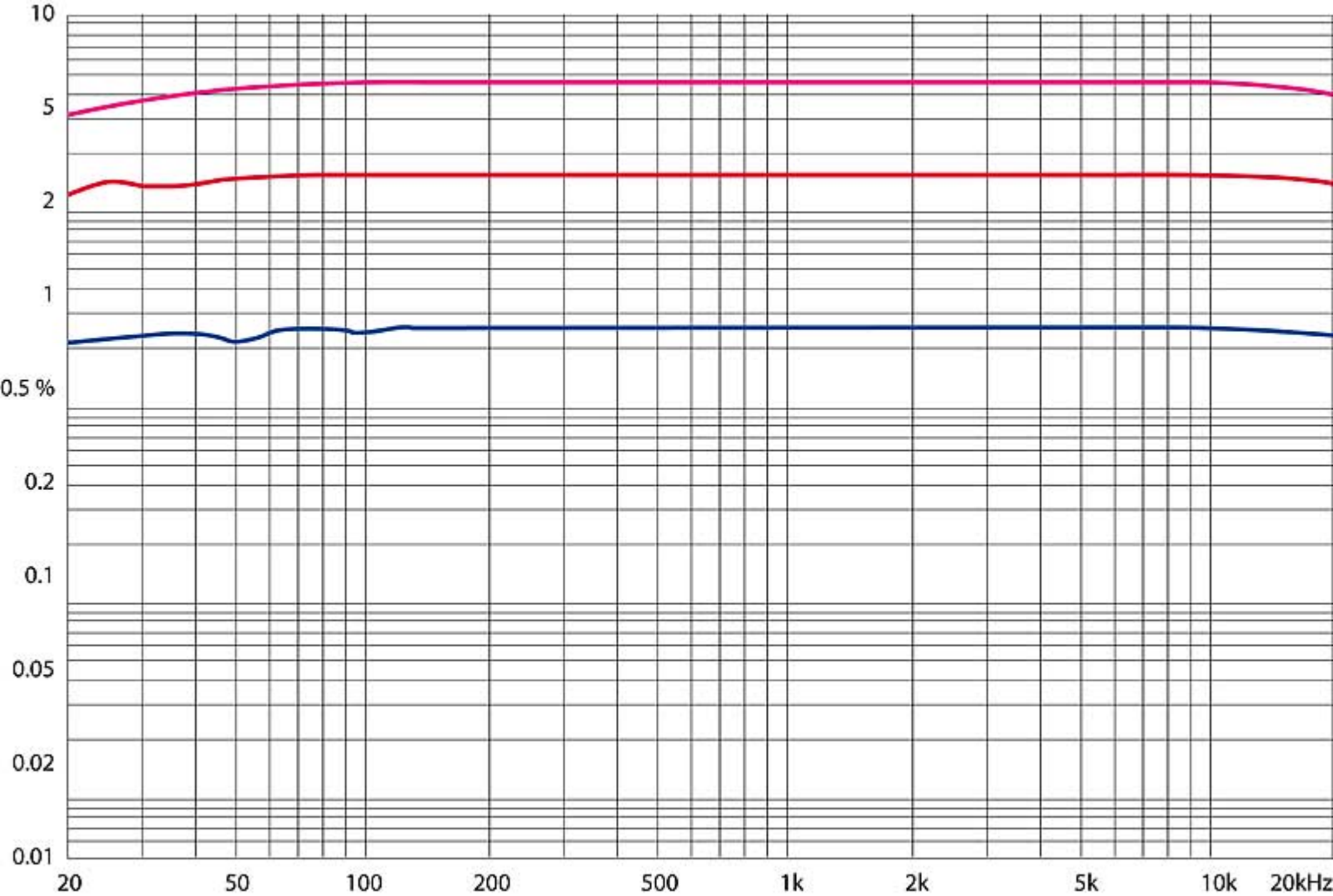
DISTORSIONE ARMONICA / RISPOSTA IN FREQUENZA @ 1 - 20 - 40 W su 4ohm
