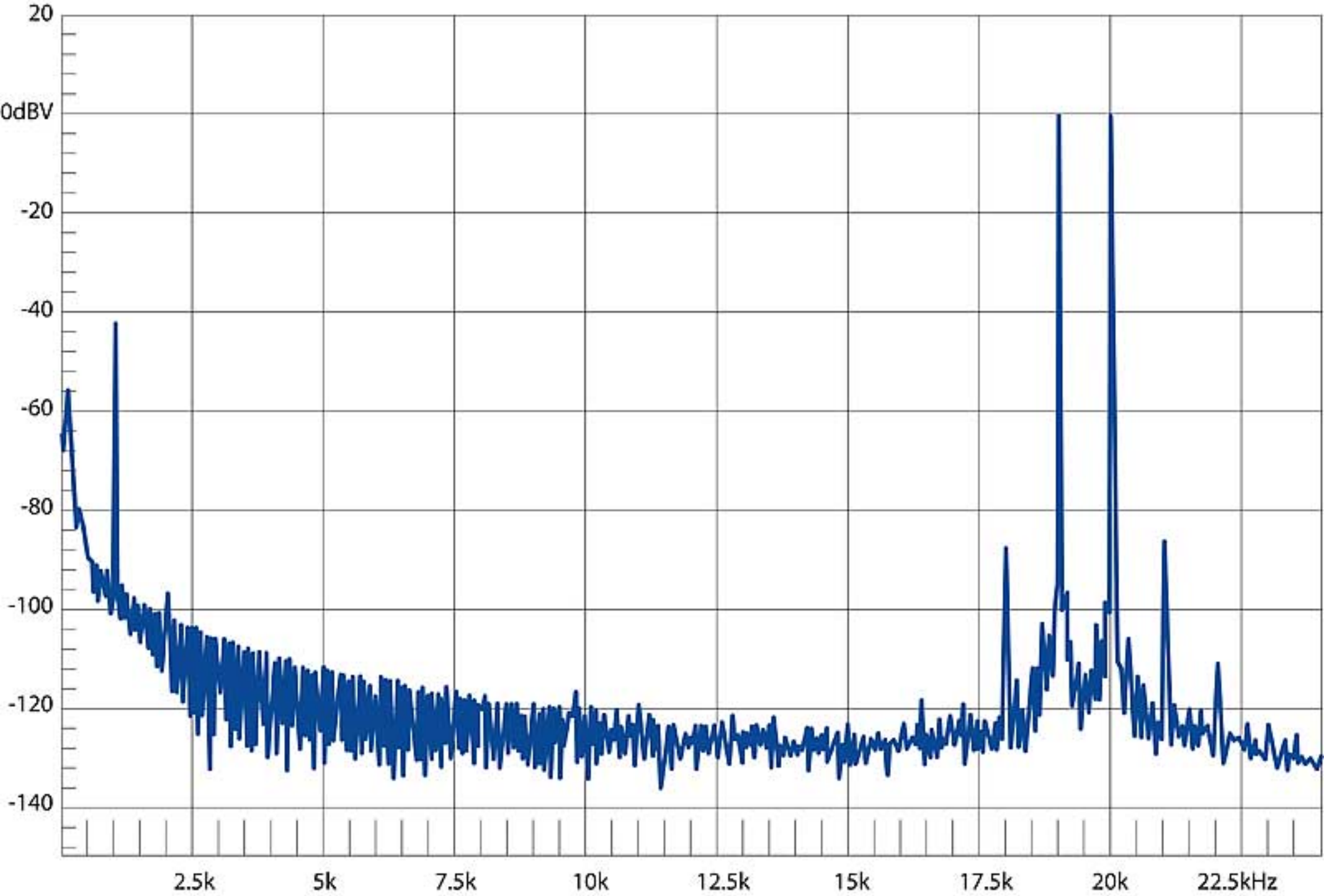
ANALISI DI SPETTRO IN FFT 19 E 20k Hz A 1 watt SU 4 ohm
