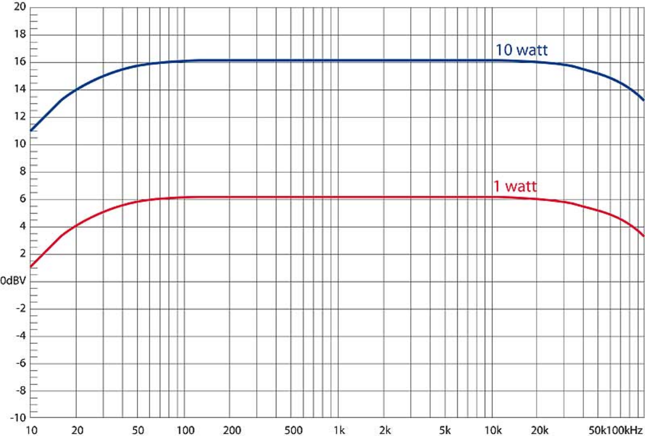
RISPOSTA IN FREQUENZA A 1 watt E 10 watt SU 4 ohm
