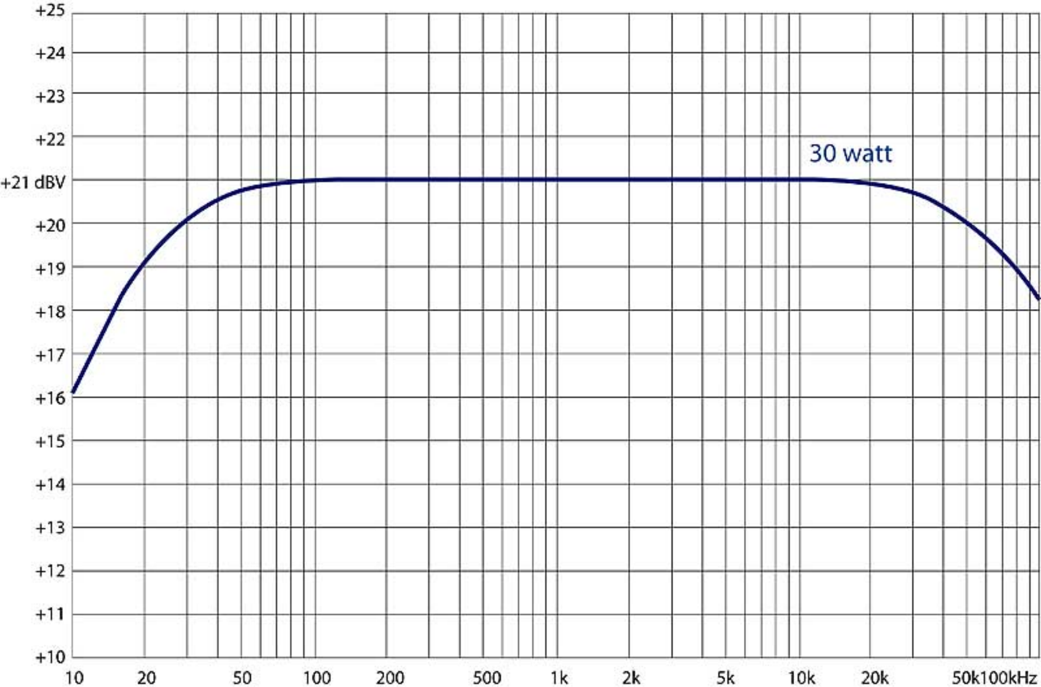
RISPOSTA IN FREQUENZA A 30 watt SU 4 ohm
