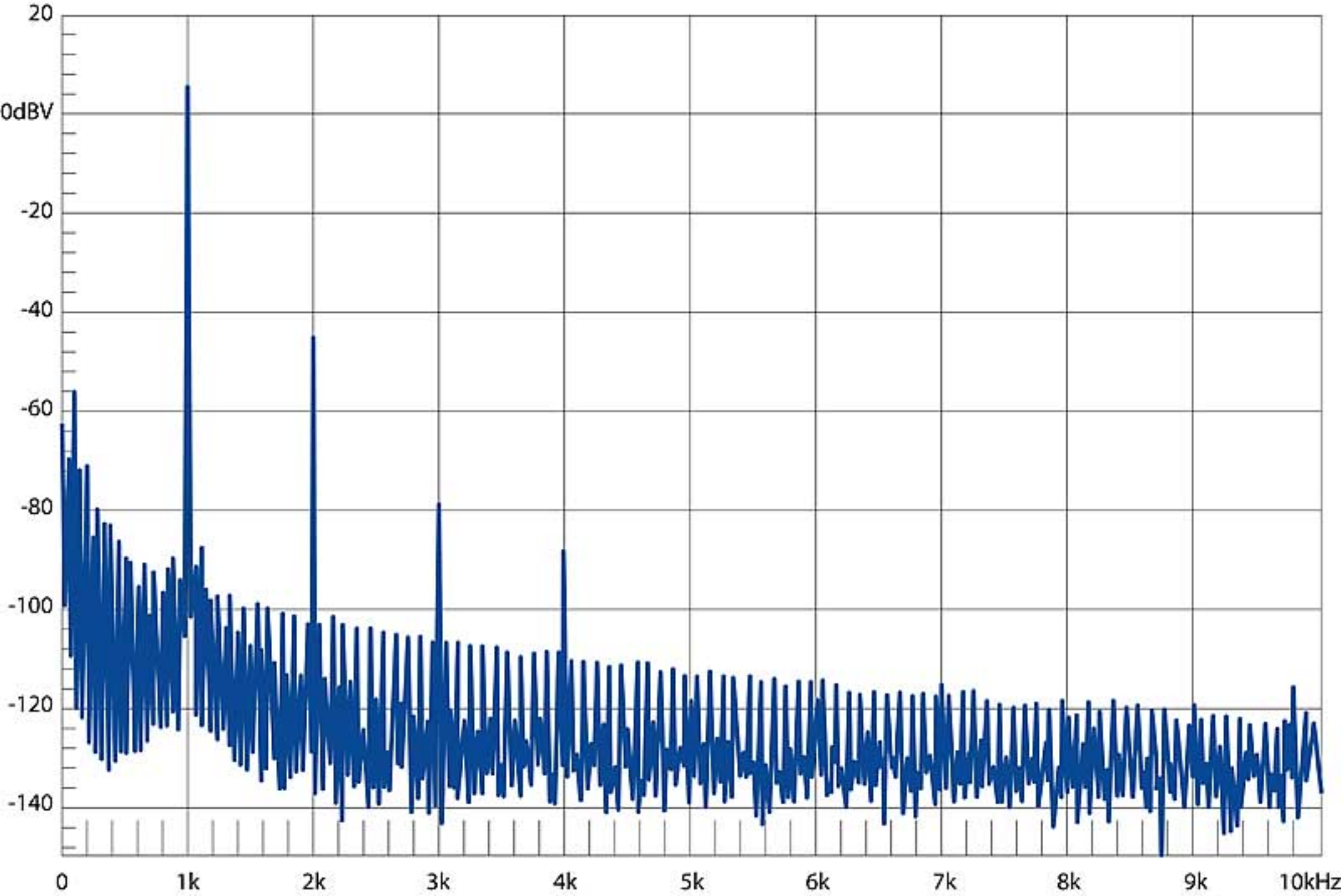
ANALISI DI SPETTRO IN FFT 1k Hz A 1 watt SU 4 ohm
