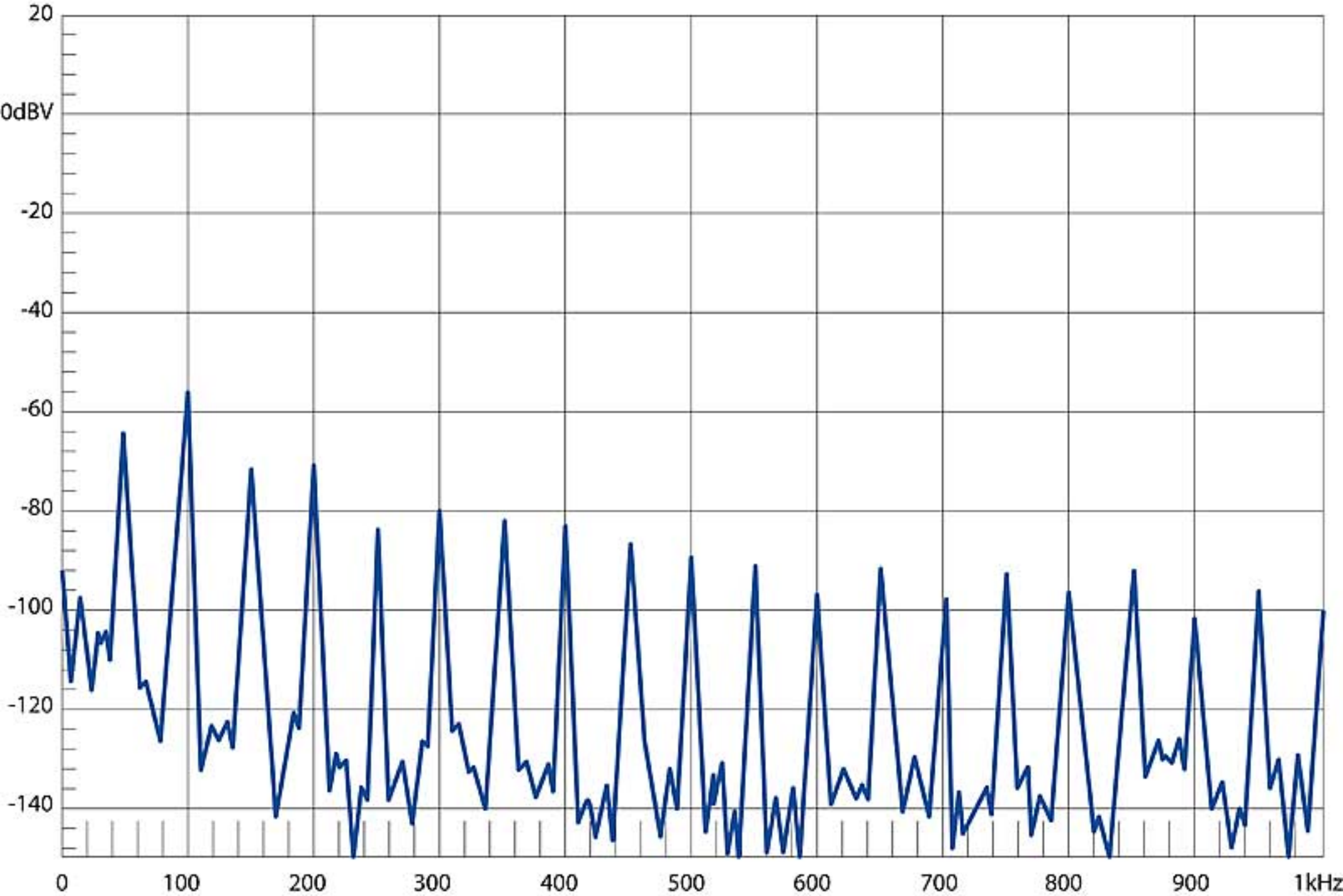
ANALISI DI SPETTRO IN FFT SENZA INGRESSO A 1 watt SU 4 ohm
